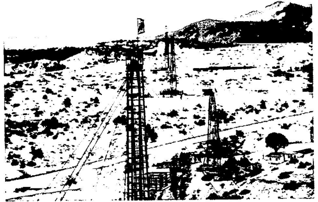
土耳其贝帕扎里天然碱矿水平井对接工程外景
