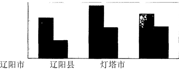
辽阳地区年日照时数直方图
